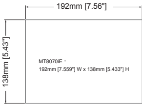
Cutout Dimensions
