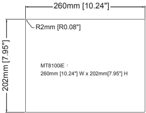
Cutout Dimensions
