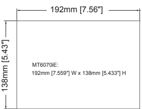
Cutout Dimensions
